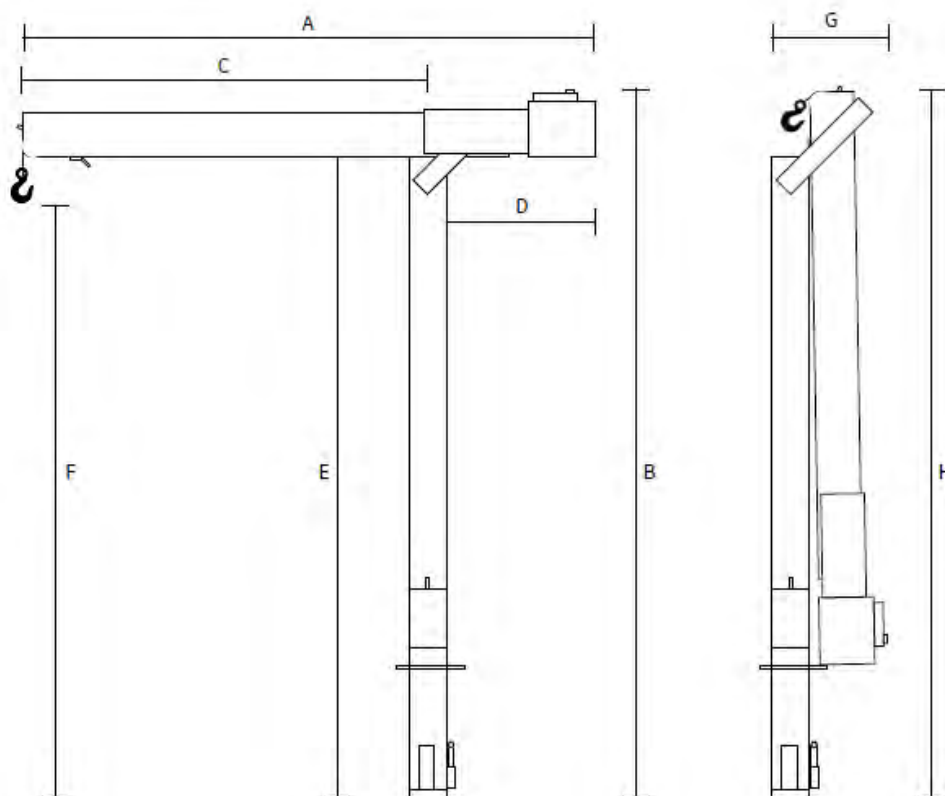
Figur 2. Tekniske specifikationer
